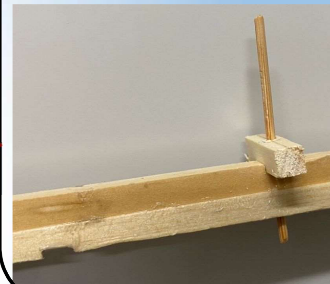
竹串を使った接合方法
