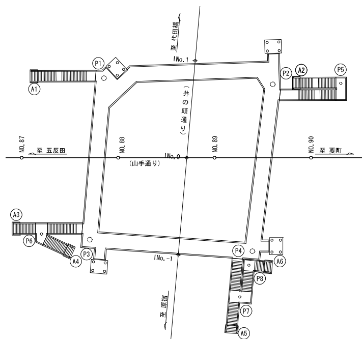
(a) 平面図
