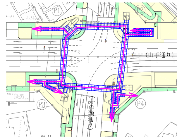
図-8 ステップ-6 (P3-P4 通路桁撤去, 新設 P3-P4 供用)
