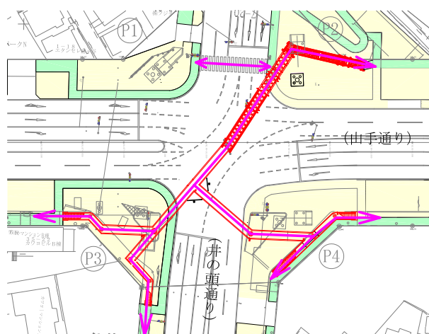
図-5 ステップ-3 (P1 通路析撤去)
