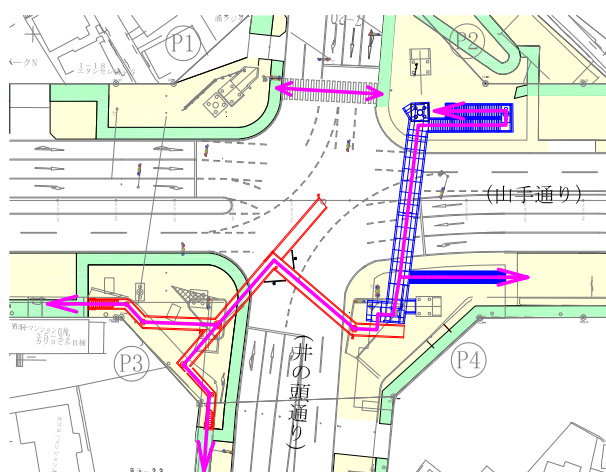
図-6 ステップ-4（新設 P2-P4 供用，P2 通路桁撤去）
