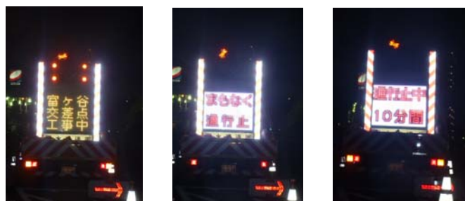
写真-1 大型LED式昇降架台広報車
