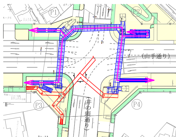
図-7 ステップ-5（新設 P1-P2, P1-P3 供用）
