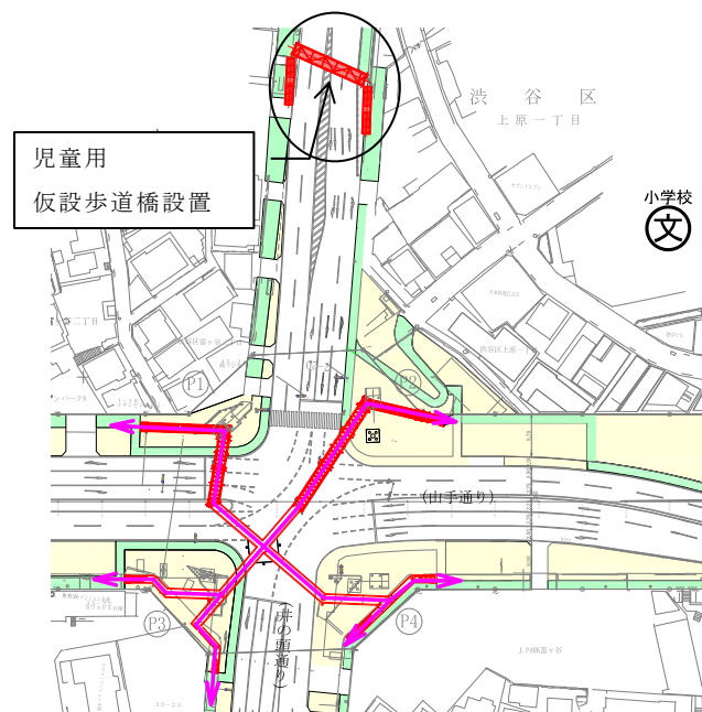
図-4 ステップ-2（通学路確保）
