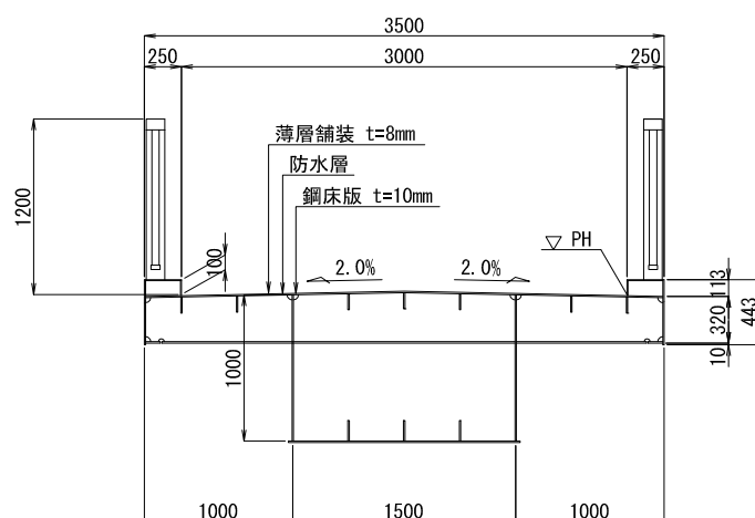
(b) 断面図
