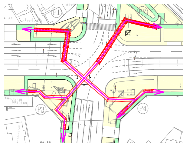
図-3 ステップ-1（施工前状況）
