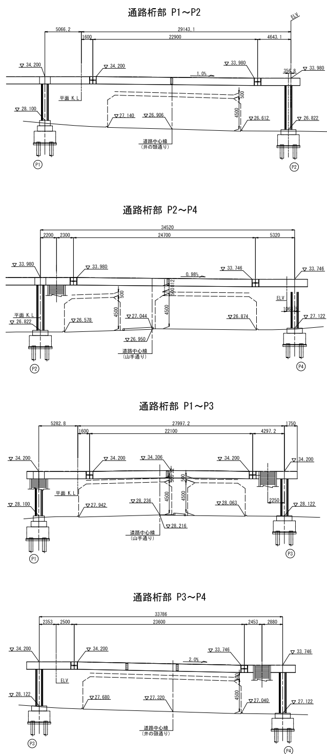
(c) 側面図
